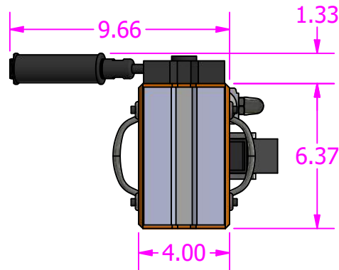
VIEW A-A
