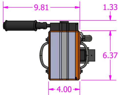
VIEW A-A
